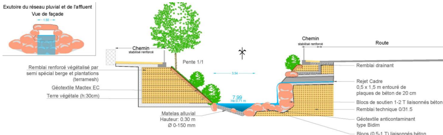
Profil en travers n° 1 : Talus renforcé végétalisé (Terramesh®) en rive gauche et aménagement de l'exutoire EP en rive droite
