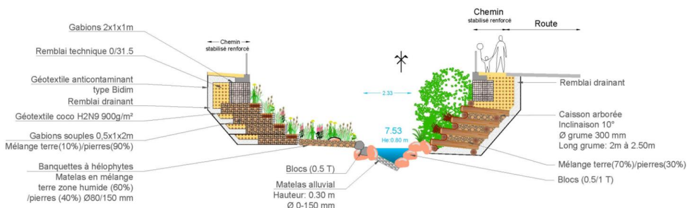
Profil en travers n°3 : Gabions souples à géonattes d'hélophytes en rive gauche et caissons végétalisés en rive droite
